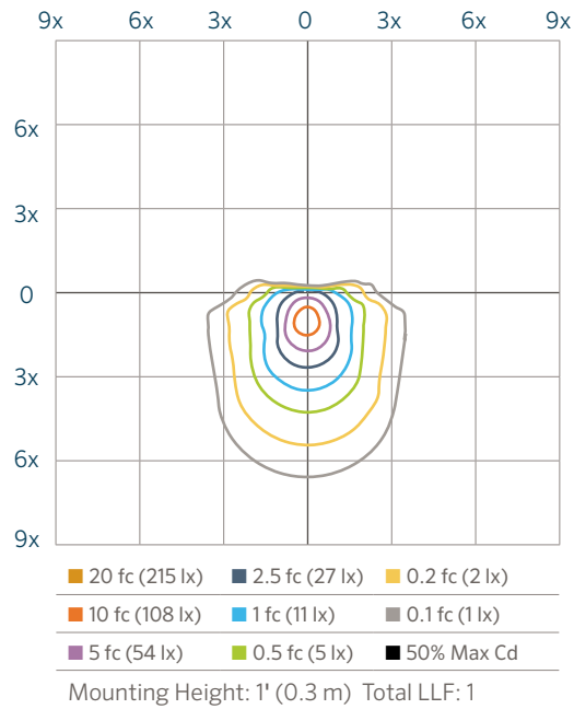
rHatch-8 ZDC Isofootcandle Plot
