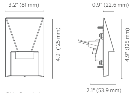
BV - Beveled
