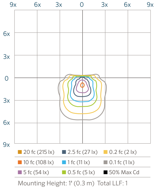
rHatch-8 1LED Isofootcandle Plot
